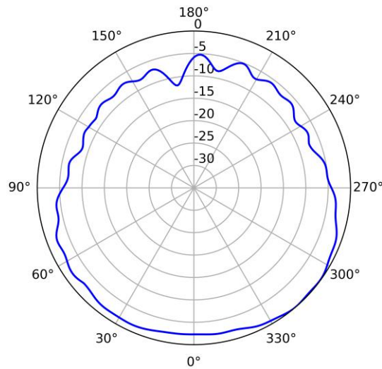
2.4GHz (Vertical)
